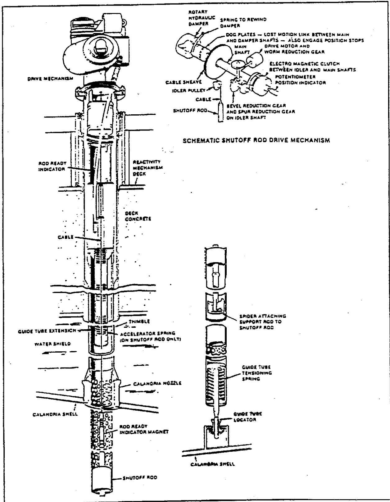
Figure 6.6 Barre d'arrêt.
